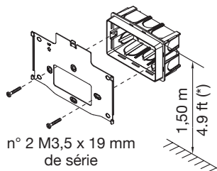
Boîtier Mod.503
